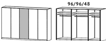
250cm 5 door 1 mirror robe W 250 X D 58 X H 216 cm
