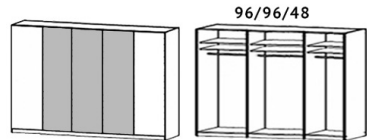
250cm 5 door 3 mirror robe W 250 X D 58 X H 216 cm
