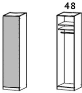
50cm 1 door 1 mirror robe W 50 X D 58 X H 216 cm
