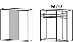
3 door 1 mirror robe W 150 X D 58 X H 220 cm
