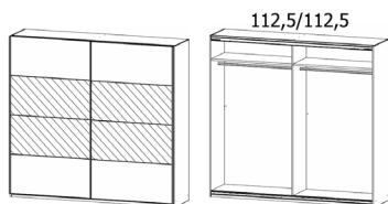
2 Door Sliding robe W 226 X D 62 X H 210 cm
