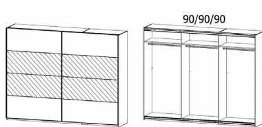
2 Door Sliding robe W 271 X D 62 X H 210 cm
