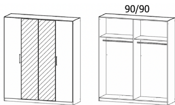
4 Door Hinged Robe W 181 X D 54 X H 210 cm
