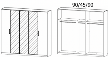
5 Door Hinged Robe W 226 X D 54 X H 210 cm
