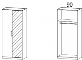
2 Door Hinged Robe W 91 X D 54 X H 210 cm
